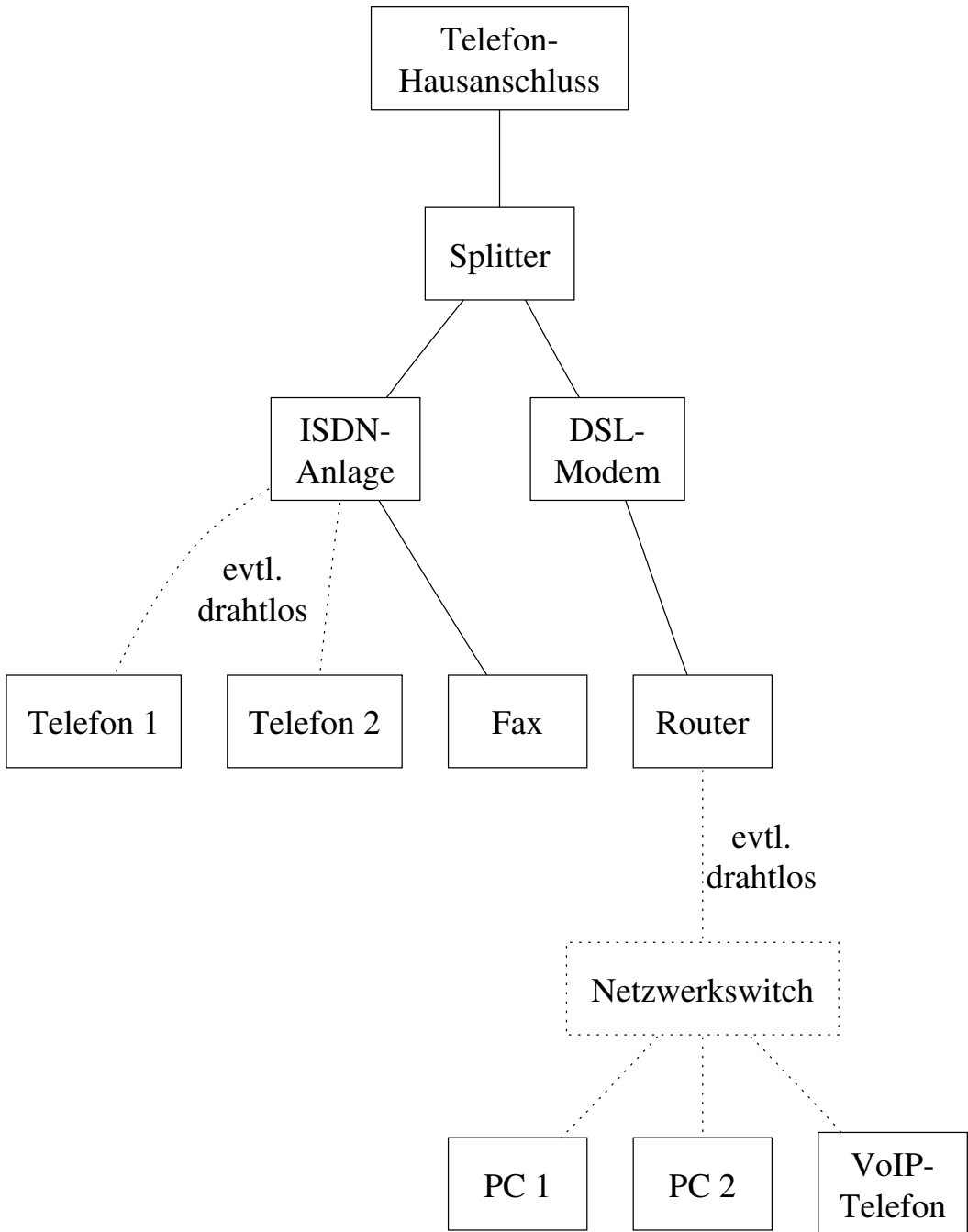
Beispiel f. DSL mit Analog-Telefon
